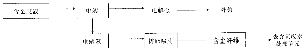
图 2-3 含金廢液電解回收金工藝流程
