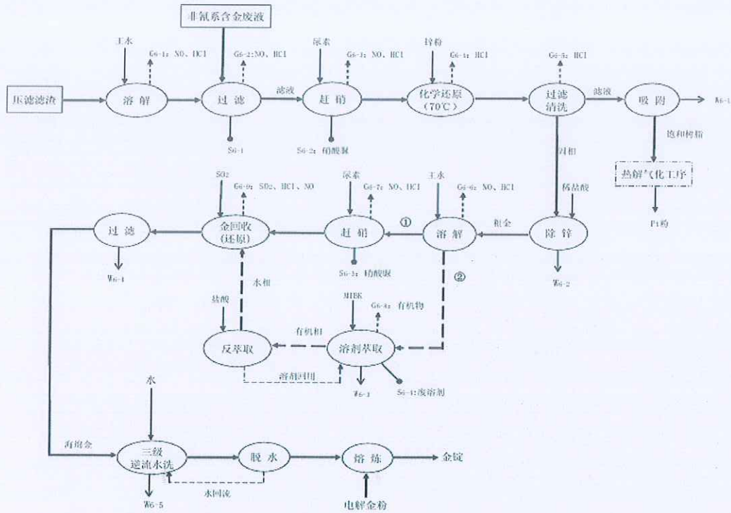
图 4.5-6-b 金回收工艺流程及产污环节
