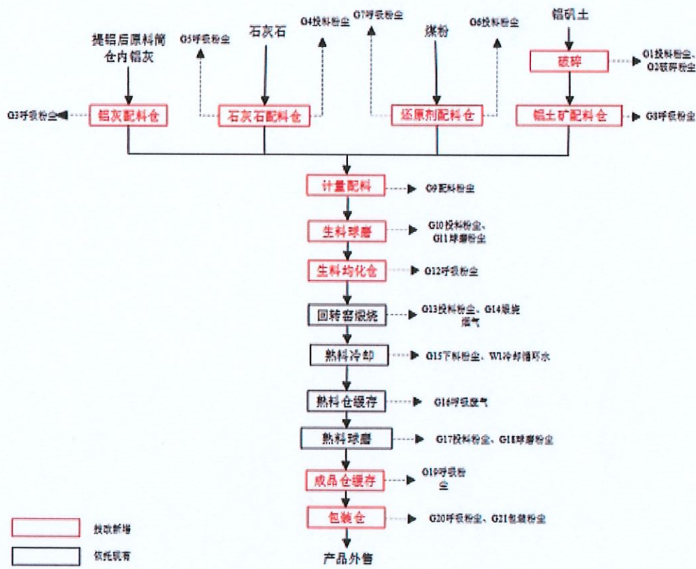
图 3.2-1 铝酸钙粉生产工艺流程图
