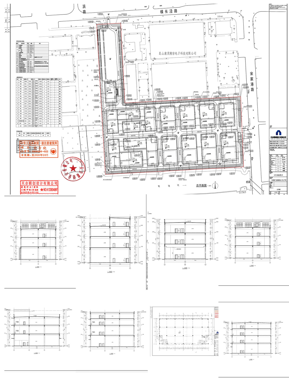
变更前的总平面图及剖面图：
