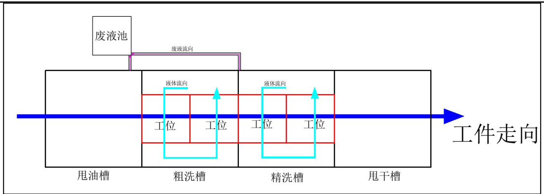
图 2-1 清洗机示意图
