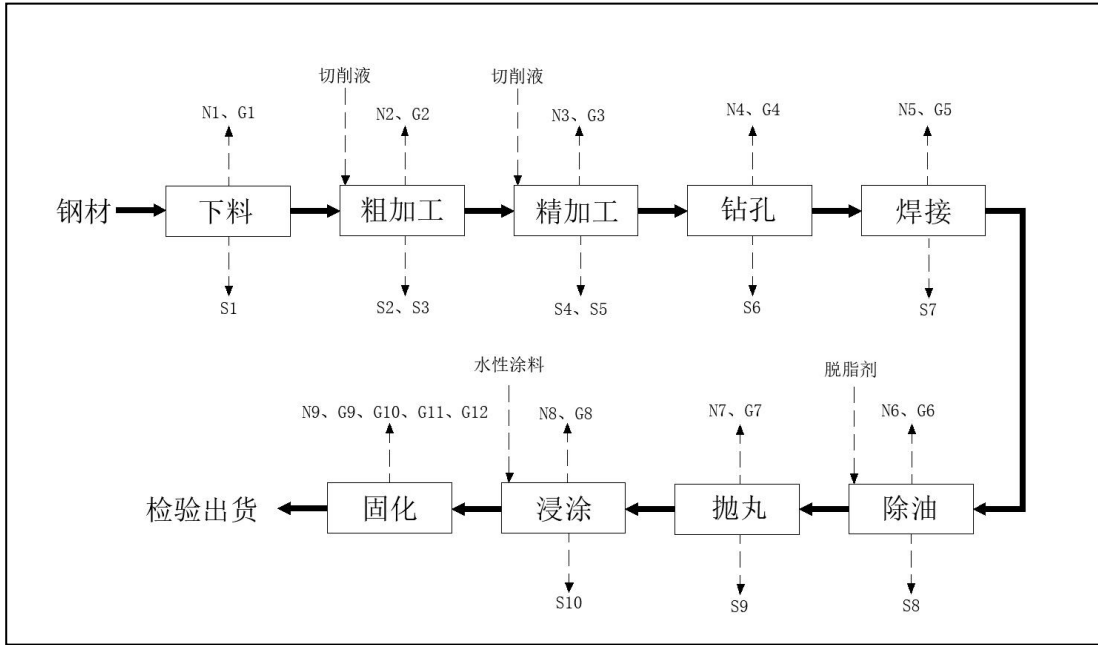
图 2-3 本项目生产工艺流程图
